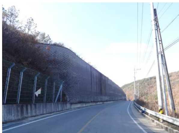
블럭식옹벽04
